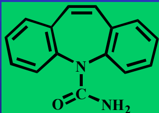
Carbamazepin
