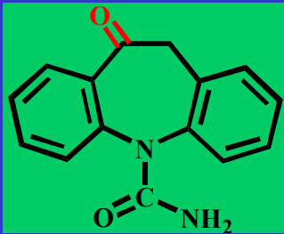
Oxcarbazepin
