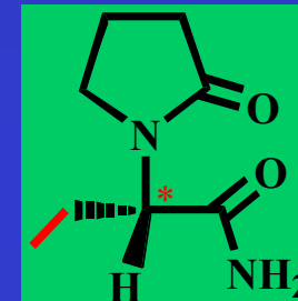
Levetiracetam
